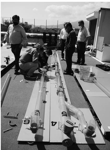
内部が見えるよう透明管を使った模擬配管機材
